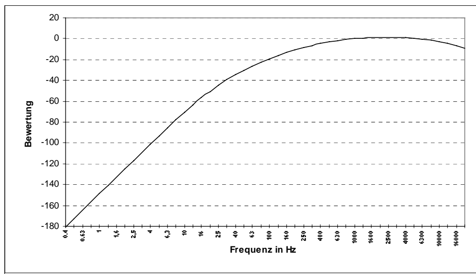
Bild 1: A-Bewertungskurve
